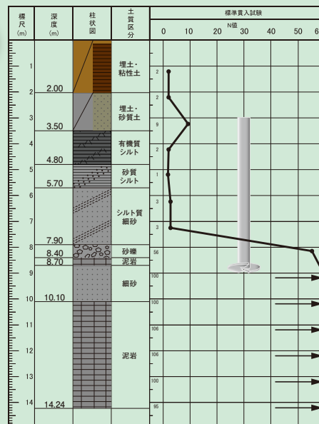
ボーリング柱状図
