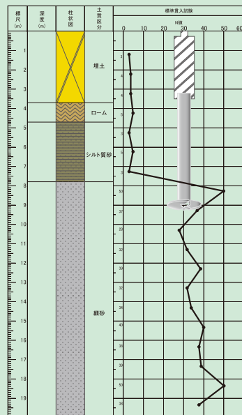
ボーリング柱状図
